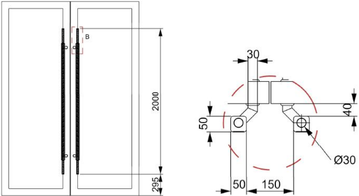
尺寸图:
