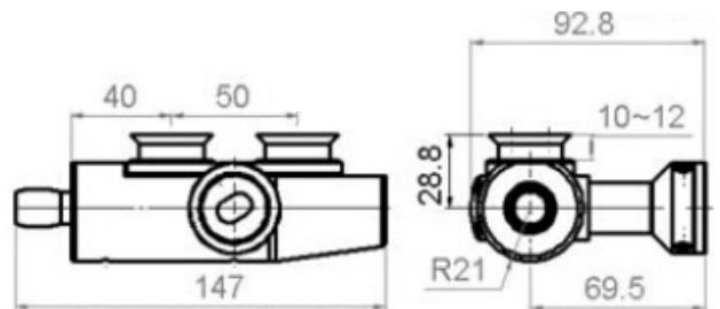
D 款：入墙顶轴+直上轴+直下轴
