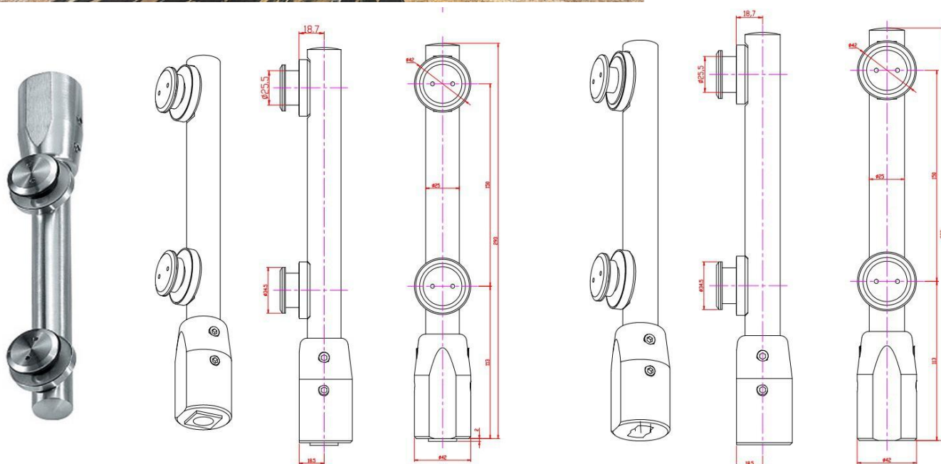
上轴（方孔）
