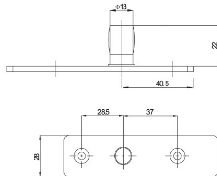
门框上轴
